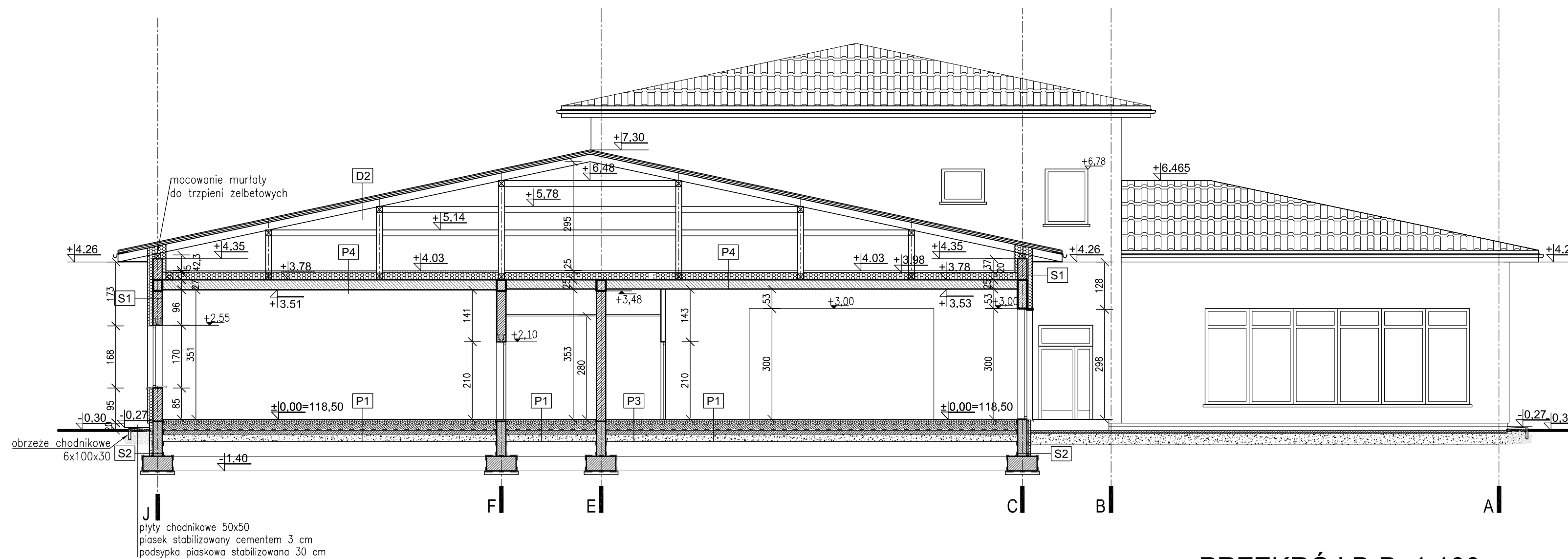
PRZEKRÓJ B-B 1:100 ELEWACJA PÓŁNOCNA 1:100
