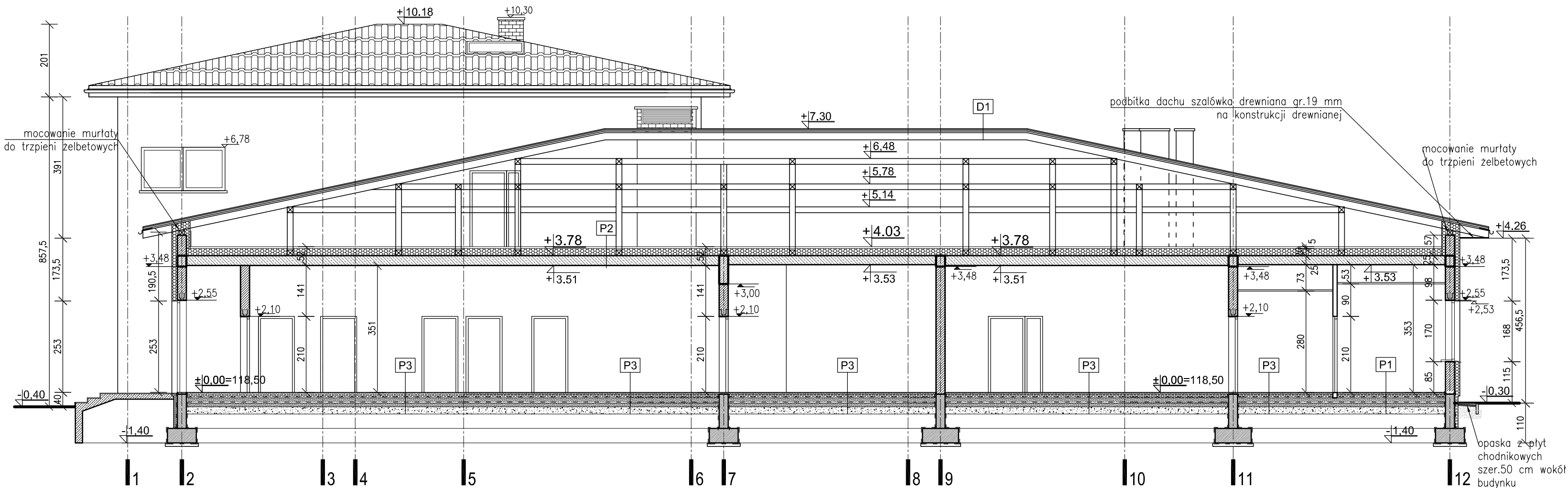
PRZEKRÓJ D-D 1:100
