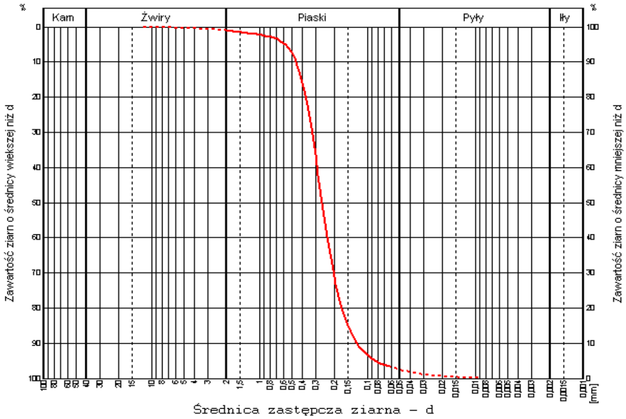
Wykres kumulacyjny próbki 16 (2,5 m)
