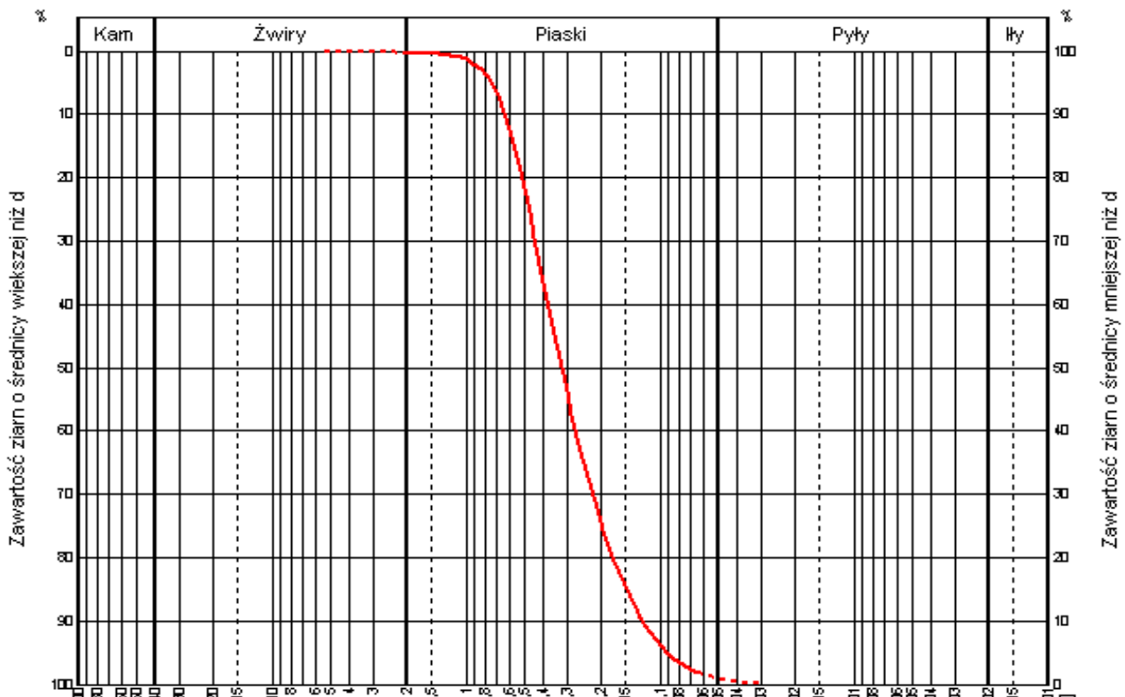
Wykres kumulacyjny próbki 16 (2,5 m)
