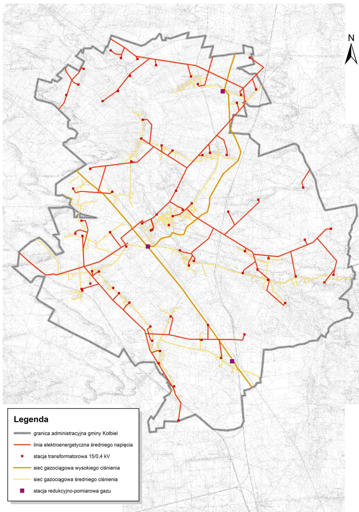
Rysunek 12. Sieci elektroenergetyczne oraz gazowe.
